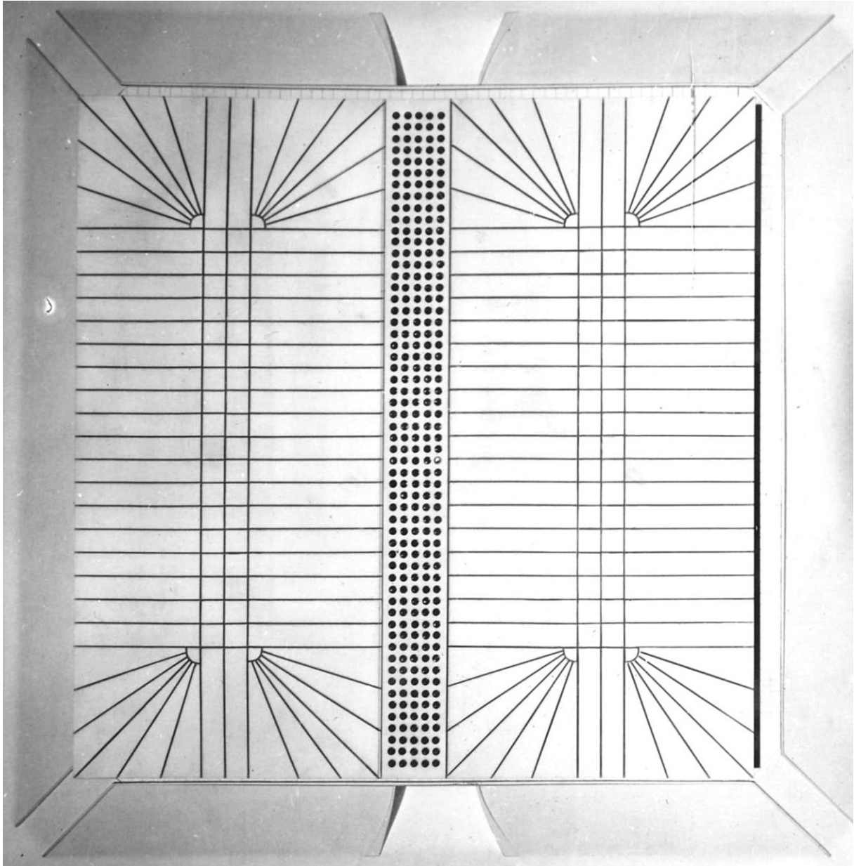
6.kép. BNV, a tetőszerkezet makettfotón. Jól látszik a két lapos „párna” és a teherhordási irányokat kirajzoló hálózat, valamint a közöttük lévő felülvilágító sáv. 6667
