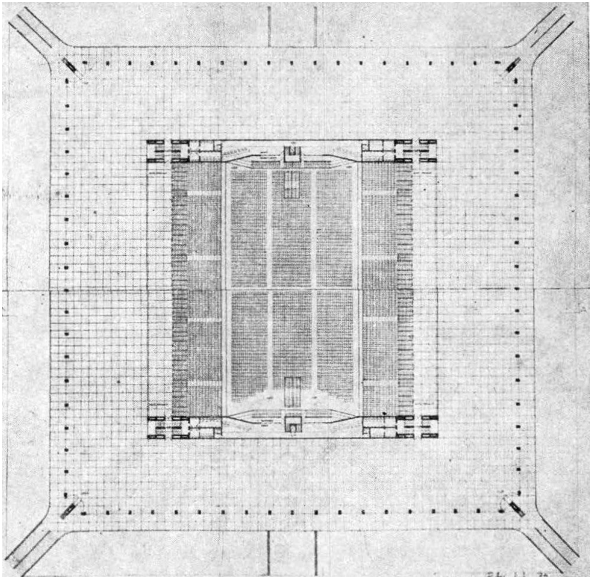
2.kép. BNV, galéria alaprajz (pályázati terv). MÉ 1963/5
