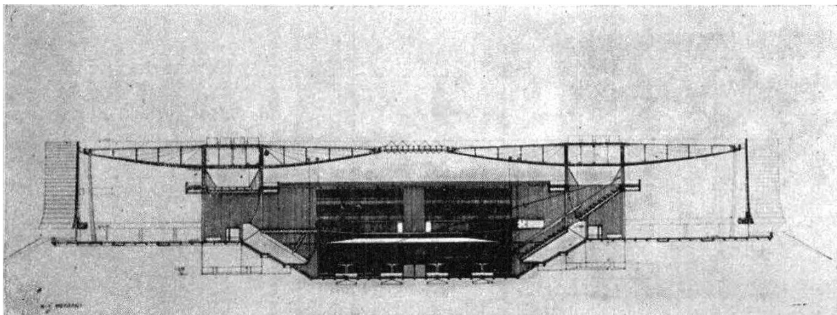
3.kép. BNV, keresztmetszet, a Dunával párhuzamosan felvéve (pályázati terv), itt még a tetőszerkezetet tartó faltestbe integrálták a VIP, és közvetítő helyiségcsoportot. MÉ 1963/5
